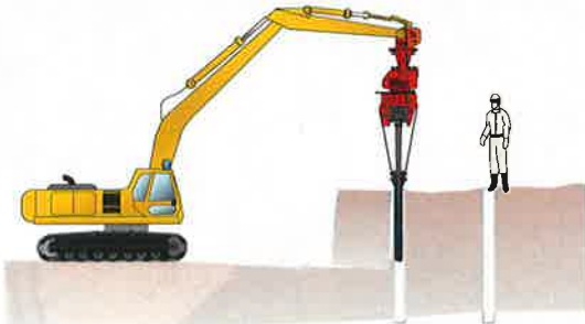
特殊くさび式割岩装置の建込
